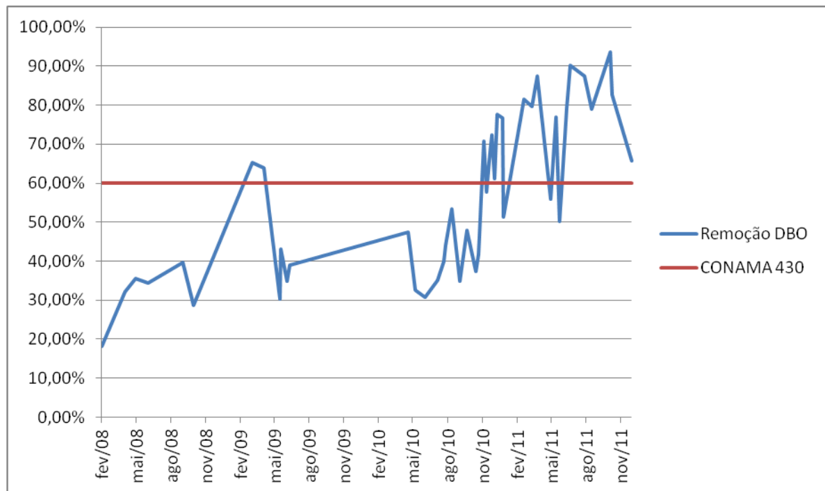
Figura 4 – Gráfico de Eficiência na remoção de DBO
