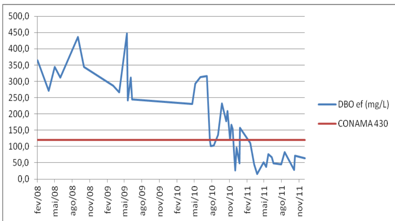
Figura 3 – Gráfico do efluente final
